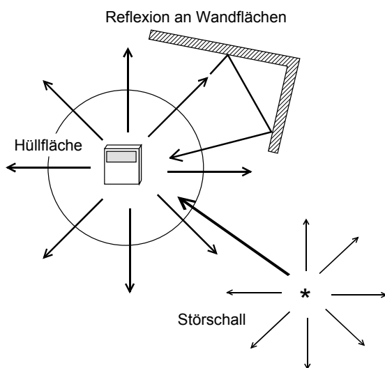
Abb. 3 Unerwünschte Anteile bei der Schallleistungsmessung mit der Schalldruckmethode: Störschall und Raumreflexionen.
