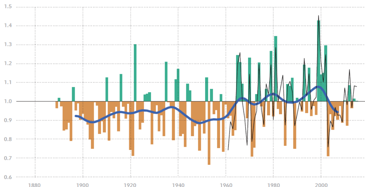
Abbildung 4: Verhältnis des Jahresniederschlags zur Norm 1961–1990 an der Station Sargans: positive Abweichungen (grün), negative (braun), geglätteter Verlauf (dicke Linie), Werte von Vaduz (dünne Linie). Quelle: AU 2016, MeteoSchweiz
