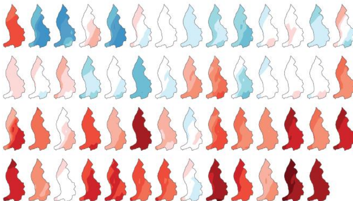
Abbildung 3: Jährliche Temperaturabweichungen vom Mittel 1961–1990 in Liechtenstein für die Jahre 1961–2015; Farbskala von -2.5 (blau) bis +2.5°C (dunkelrot). Quelle: AU 2016, MeteoSchweiz
