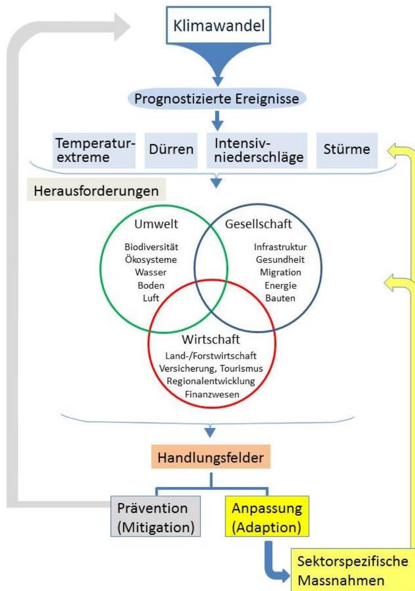
Abbildung 1: Schematische Darstellung der Zusammenhänge bedingt durch den Klimawandel.
