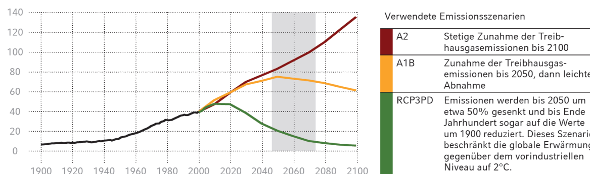
Abbildung 5: Mögliche Emissionsszenarien. Quelle: AU 2016, MeteoSchweiz
