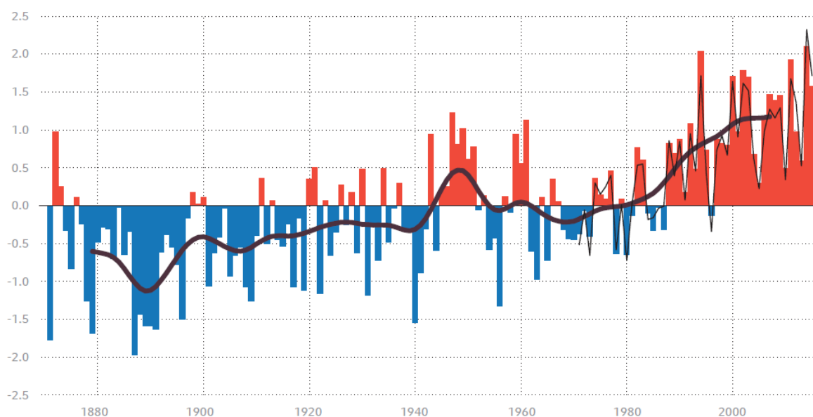
Abbildung 2: Abweichung der Jahresmitteltemperatur in Grad Celsius von der Norm 1961-1990 an der Station Bad Ragaz: positive Abweichung (rot), negative (blau), geglätteter Verlauf (dicke Linie), Werte von Vaduz (dünne Linie). Quelle: AU 2016, MeteoSchweiz
